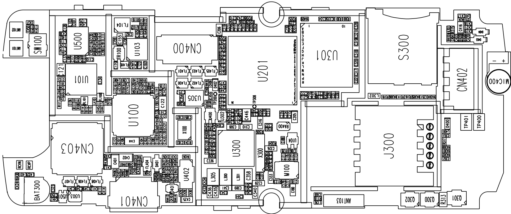
U250/KU250 - MAIN-SPF Y0147601-1.2-BTM
